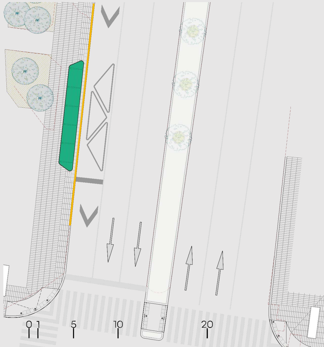
PLANTA DE CONJUNTO. NIVEL CUBIERTA
