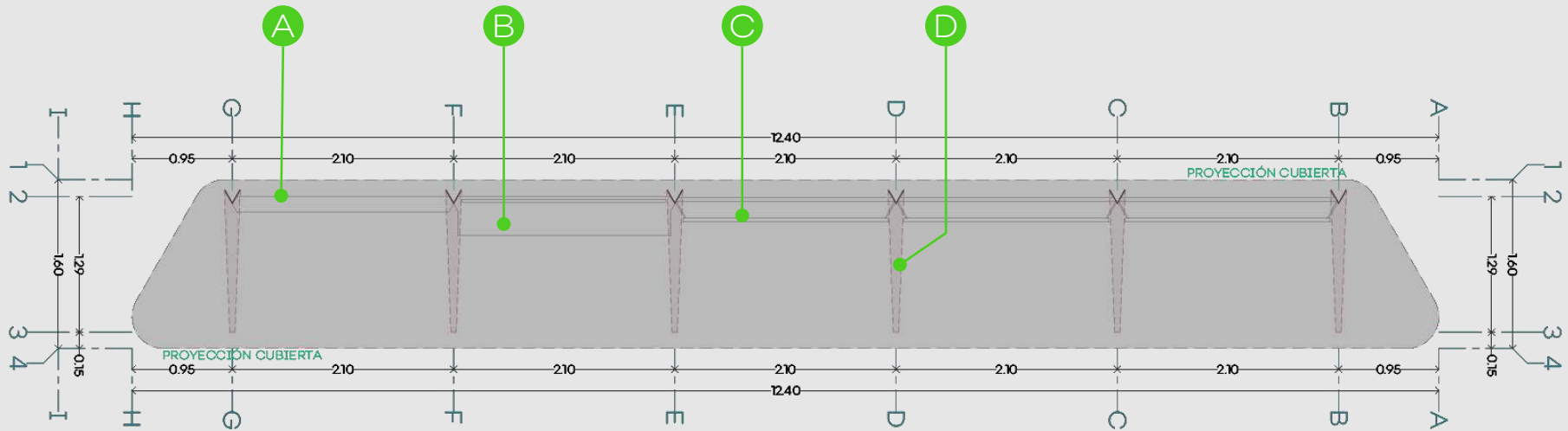
DETALLE PLANTA.
