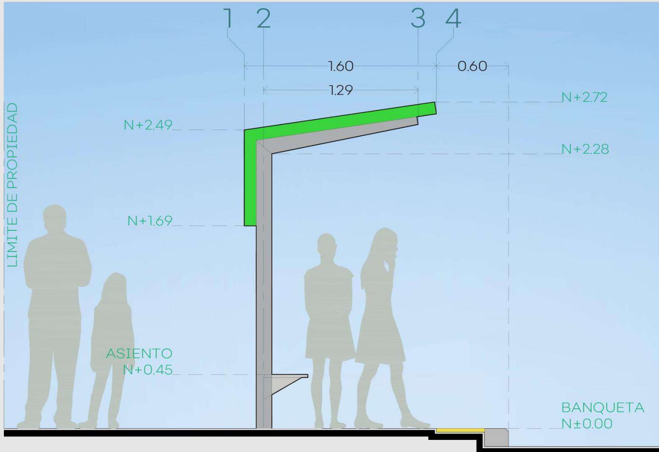
DETALLE EN SECCIÓN TRANSVERSAL
