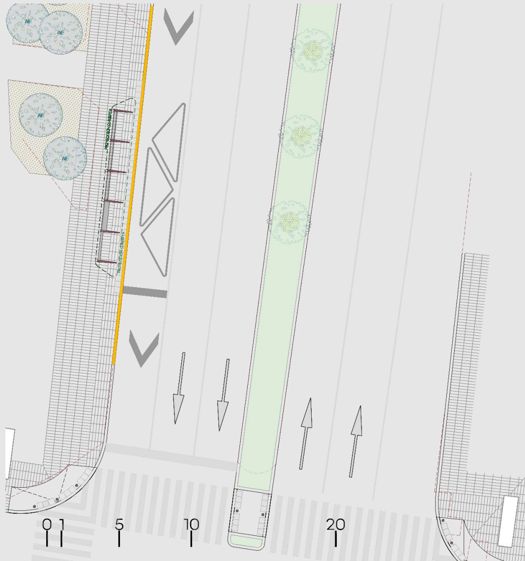
PLANTA DE CONJUNTO. NIVEL BANQUETA
